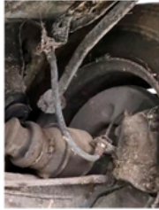
Schräglenker Gen.I, selten erhalten: Zwischenleitungen an Sätteln (104), Halter für Schlauchübergang, Verteiler+Leitung an Heckboden
